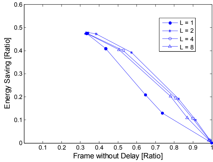
(b) NS-2
